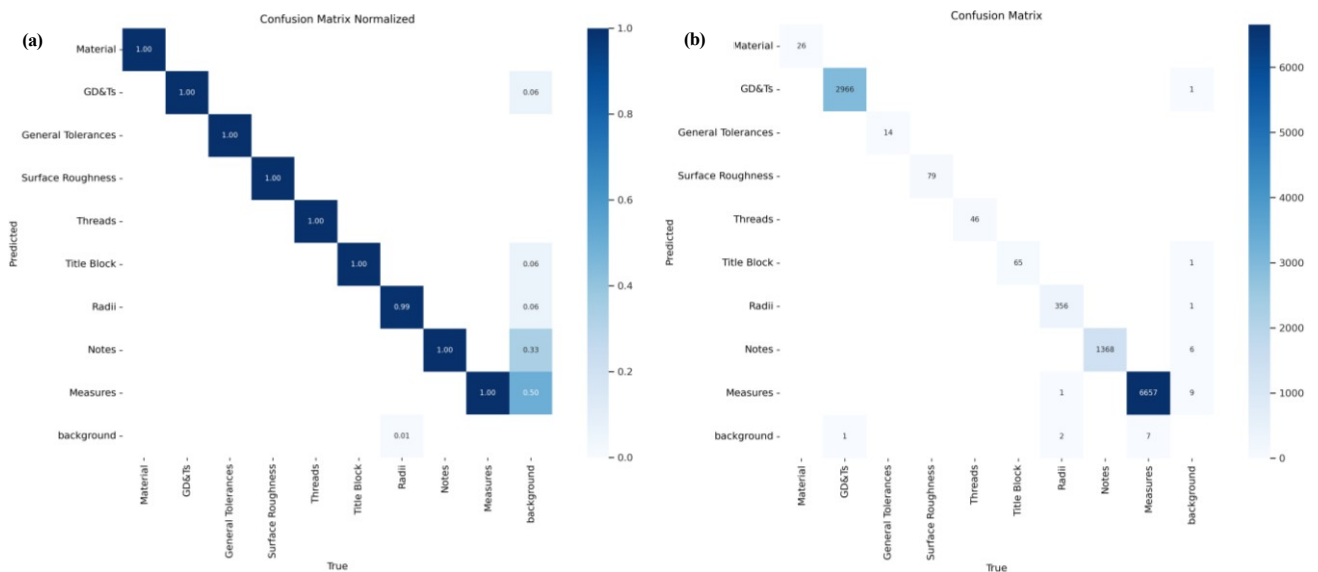
그림 13. YOLOv11-obb에 대한 혼동 행렬 평가. (a) 높은 클래스 구분 능력을 보여주는 정규화 정확도 행렬. (b) 클래스 빈도와 사소한 오분류를 보여주는 원시 예측 개수.
