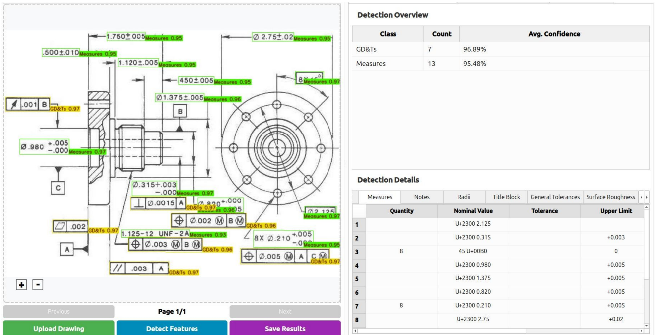
그림 A8. 회전 정보를 반영한 바운딩 박스를 사용한 YOLOv11-obb 기반 주석 위치 파악.
