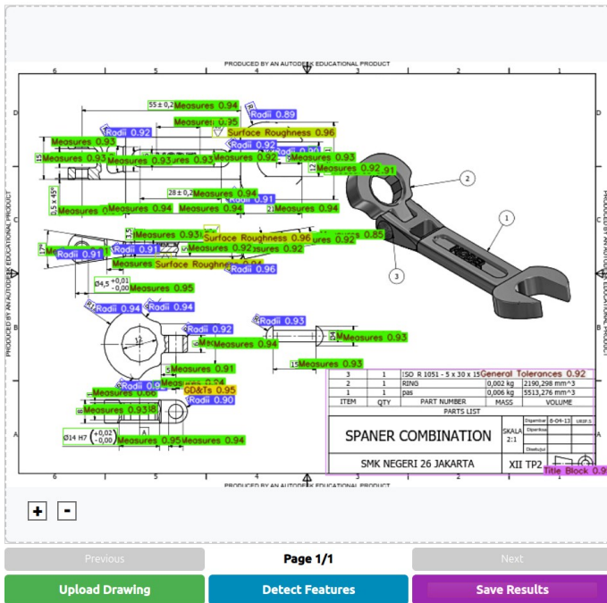
그림 A2. YOLOv11-obb를 사용하여 도면에 중첩된 탐지된 주석 영역.
